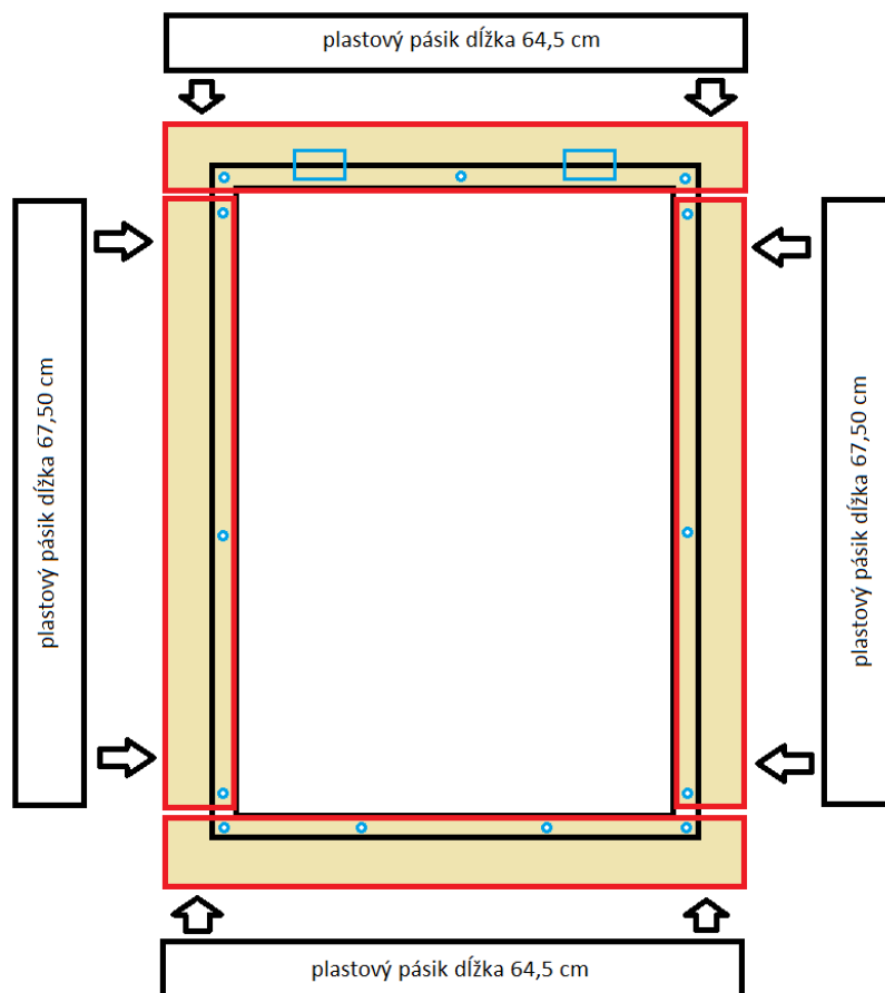
Obrázok 3 – umiestenie skrutiek
